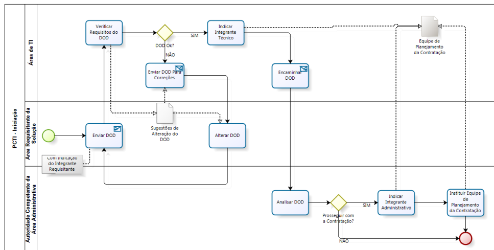
Figura 5: PCTI-P1: Iniciação
