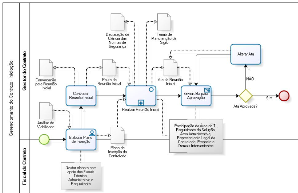
Figura 13: GCTI-P1: Iniciação
